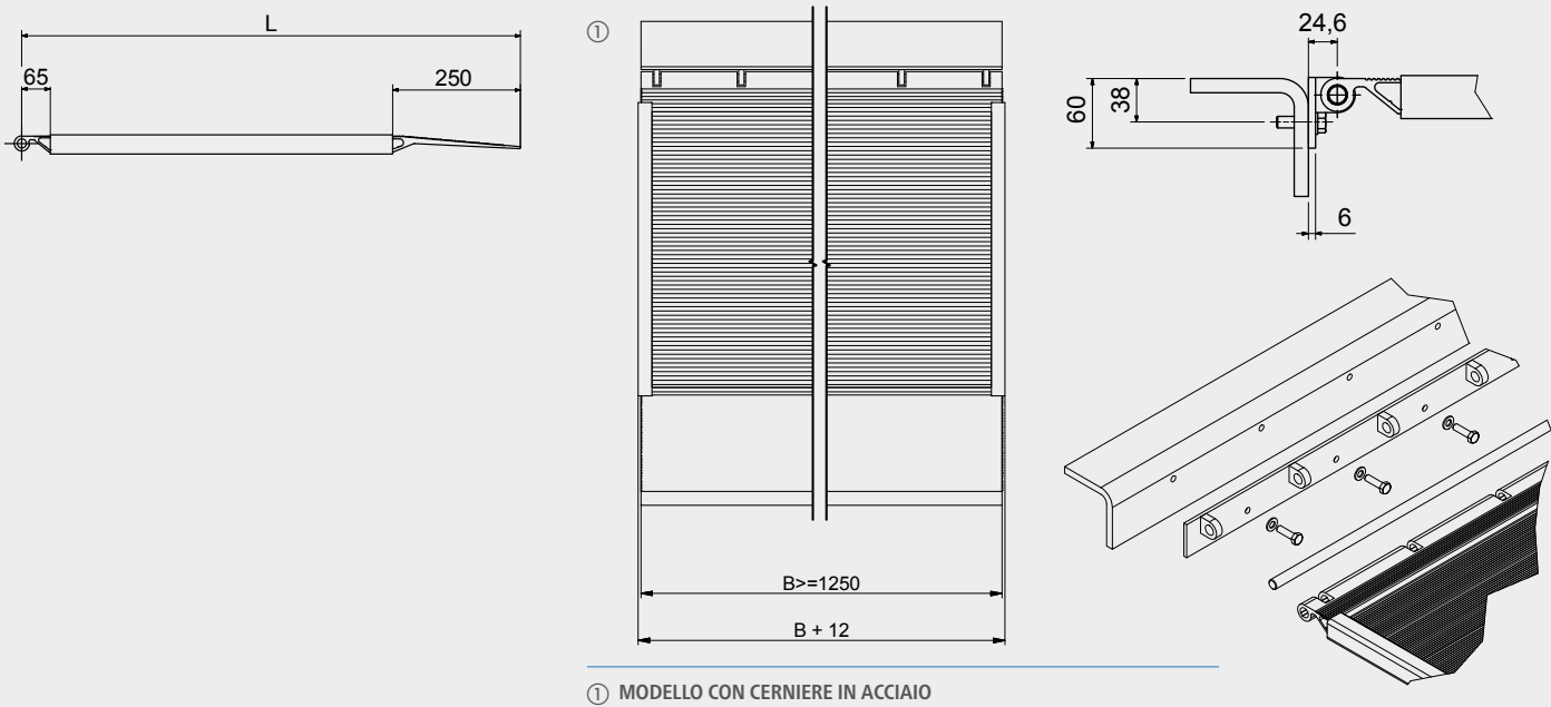
① MODELLO CON CERNIERE IN ACCIAIO
