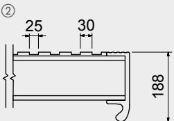
① PASSO 50/50 (STANDARD) ② PASSO SPECIALE 25/30 (SU RICHIESTA)
