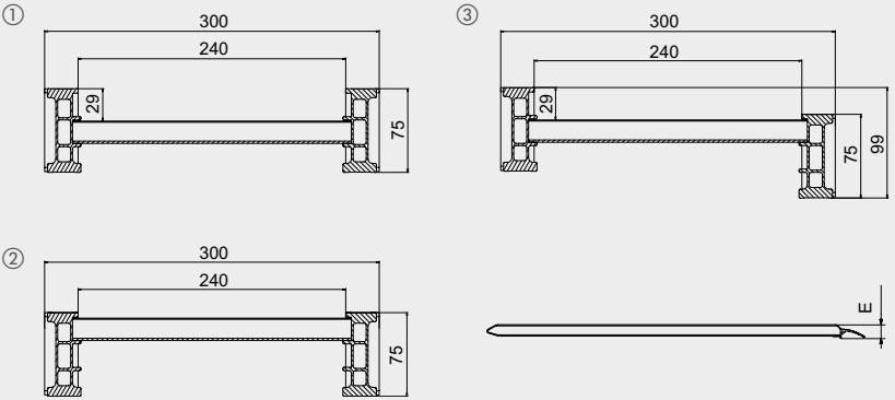
1 CON BORDI 2 SENZA BORDI 3 CON UN SOLO BORDO
