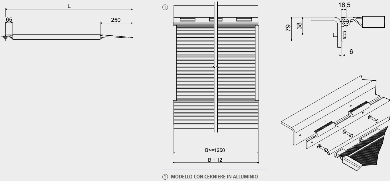
① MODELLO CON CERNIERE IN ALLUMINIO
